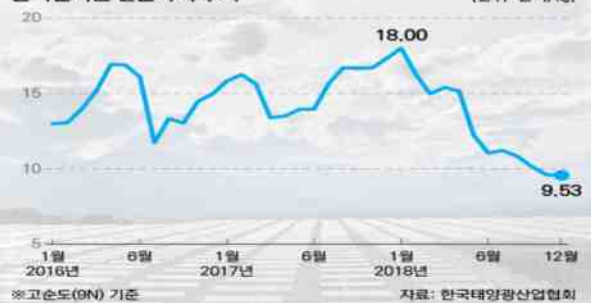
태양광 핵심소재 가격 추이
